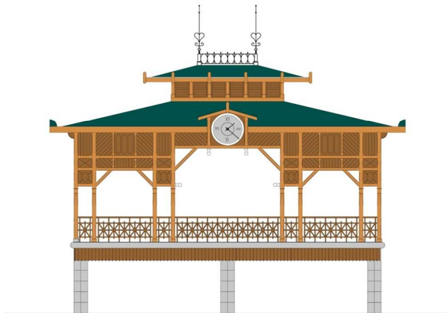
PROČELJE JUGOISTOK
